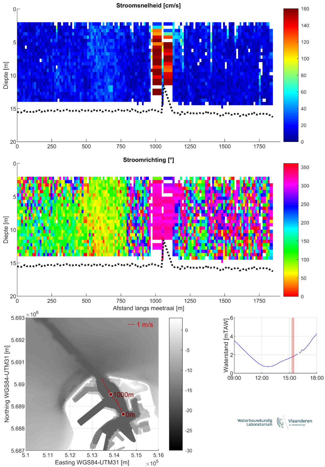
Figuur 38 – Stroomgegevens 07/08/2023 raai 33: snelheids grootte (top), -richting (midden) en diepte-gemiddelde vectoren (onder)
