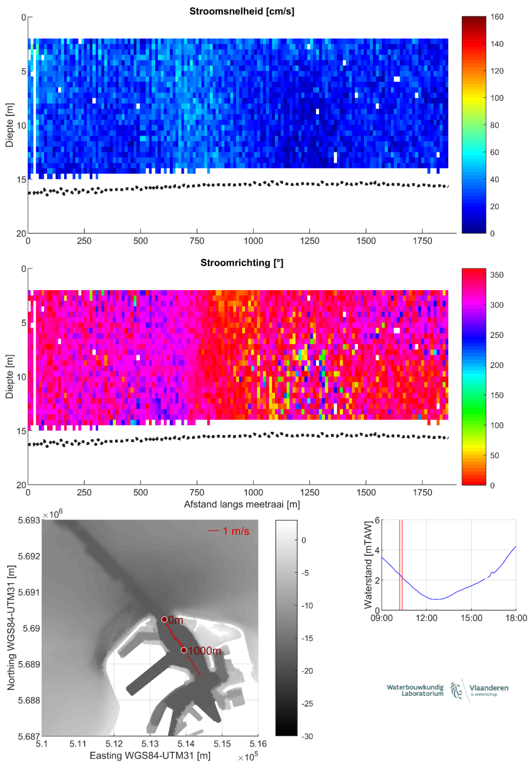
Figuur 11 – Stroomgegevens 07/08/2023 raai 6: snelheids grootte (top), -richting (midden) en diepte-gemiddelde vectoren (onder)
