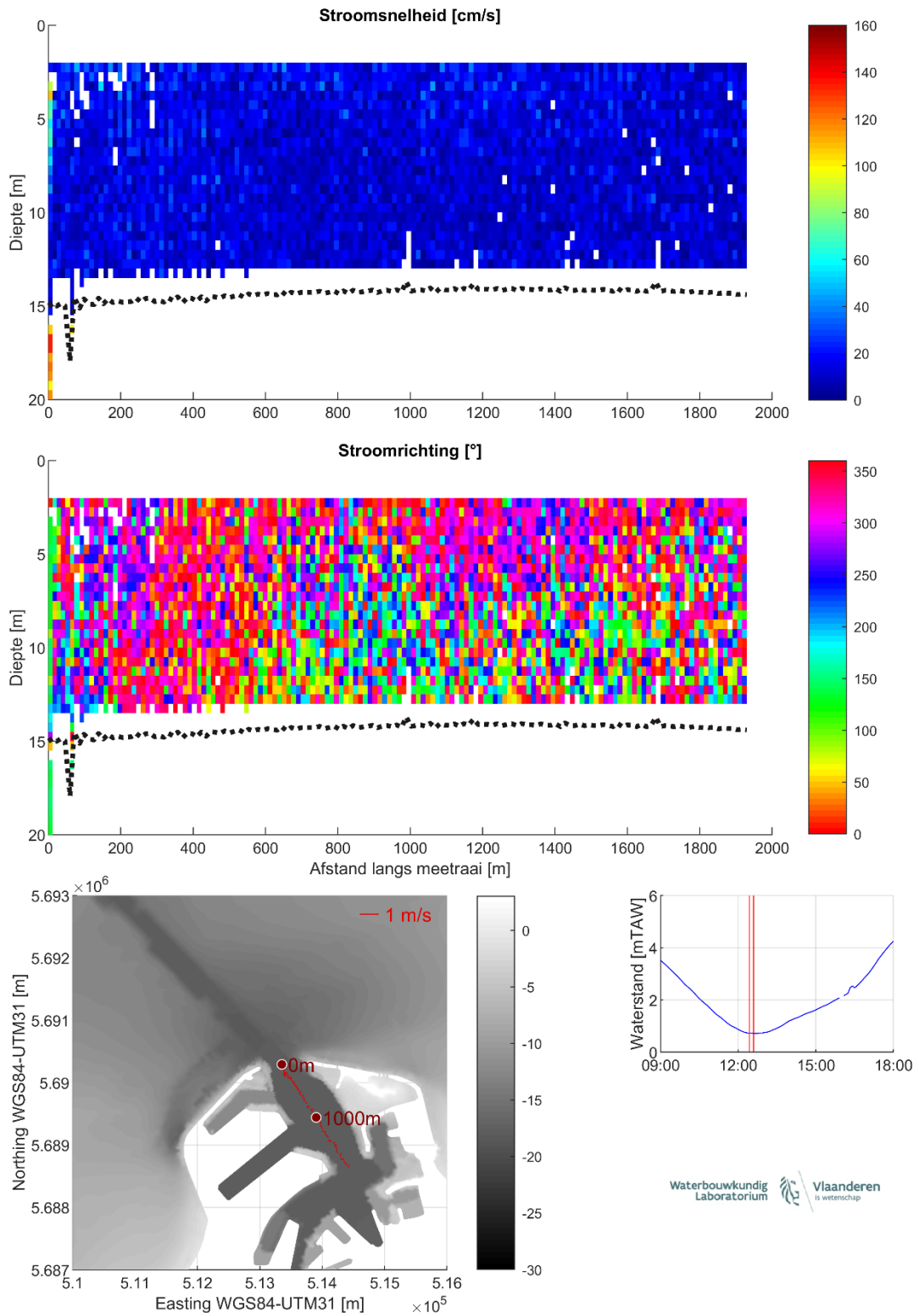
Figuur 23 – Stroomgegevens 07/08/2023 raai 18: snelheids grootte (top), -richting (midden) en diepte-gemiddelde vectoren (onder)
