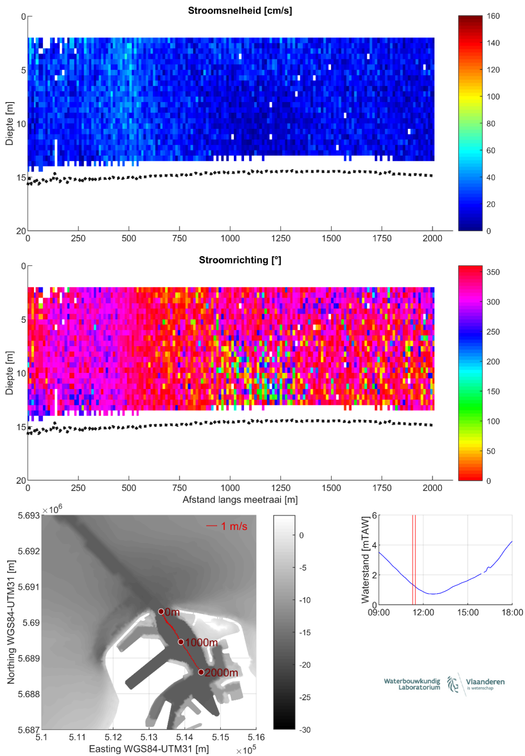
Figuur 17 – Stroomgegevens 07/08/2023 raai 12: snelheids grootte (top), -richting (midden) en diepte-gemiddelde vectoren (onder)
