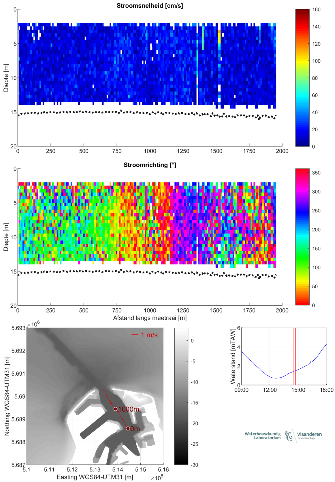
Figuur 34 – Stroomgegevens 07/08/2023 raai 29: snelheids grootte (top), -richting (midden) en diepte-gemiddelde vectoren (onder)
