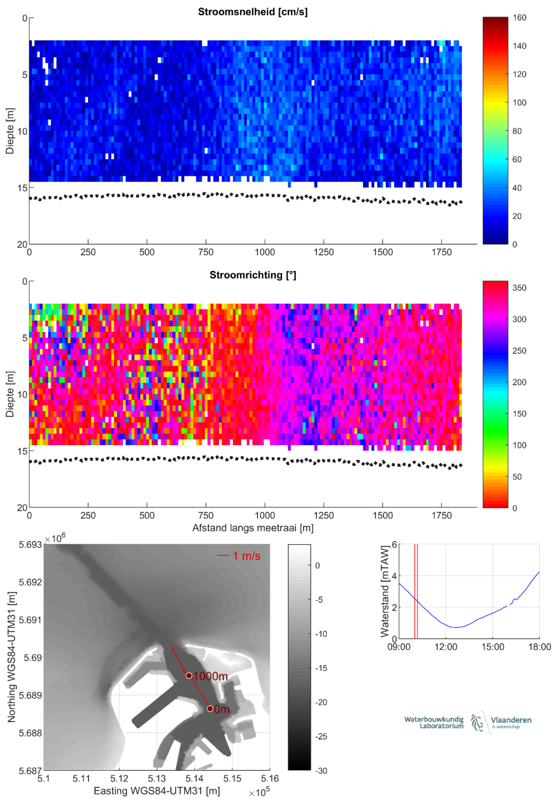
Figuur 10 – Stroomgegevens 07/08/2023 raai 5: snelheids grootte (top), -richting (midden) en diepte-gemiddelde vectoren (onder)
