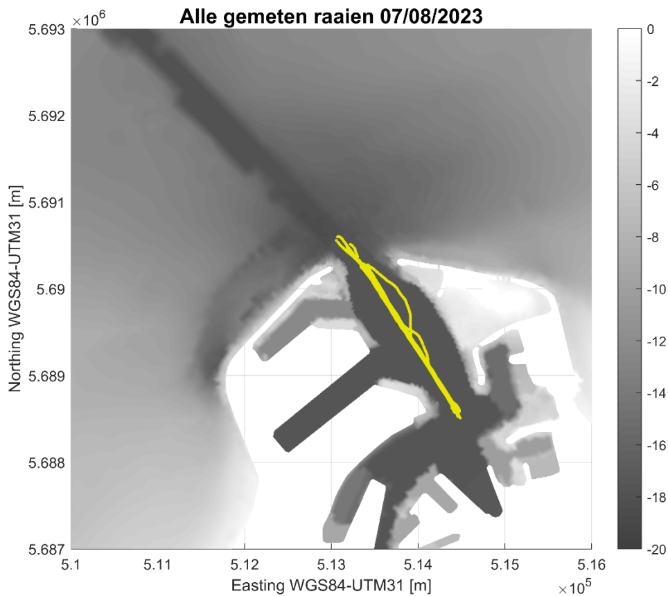
Figuur 3 – Ligging gemeten raaien op de meetdag 07/08/2023
