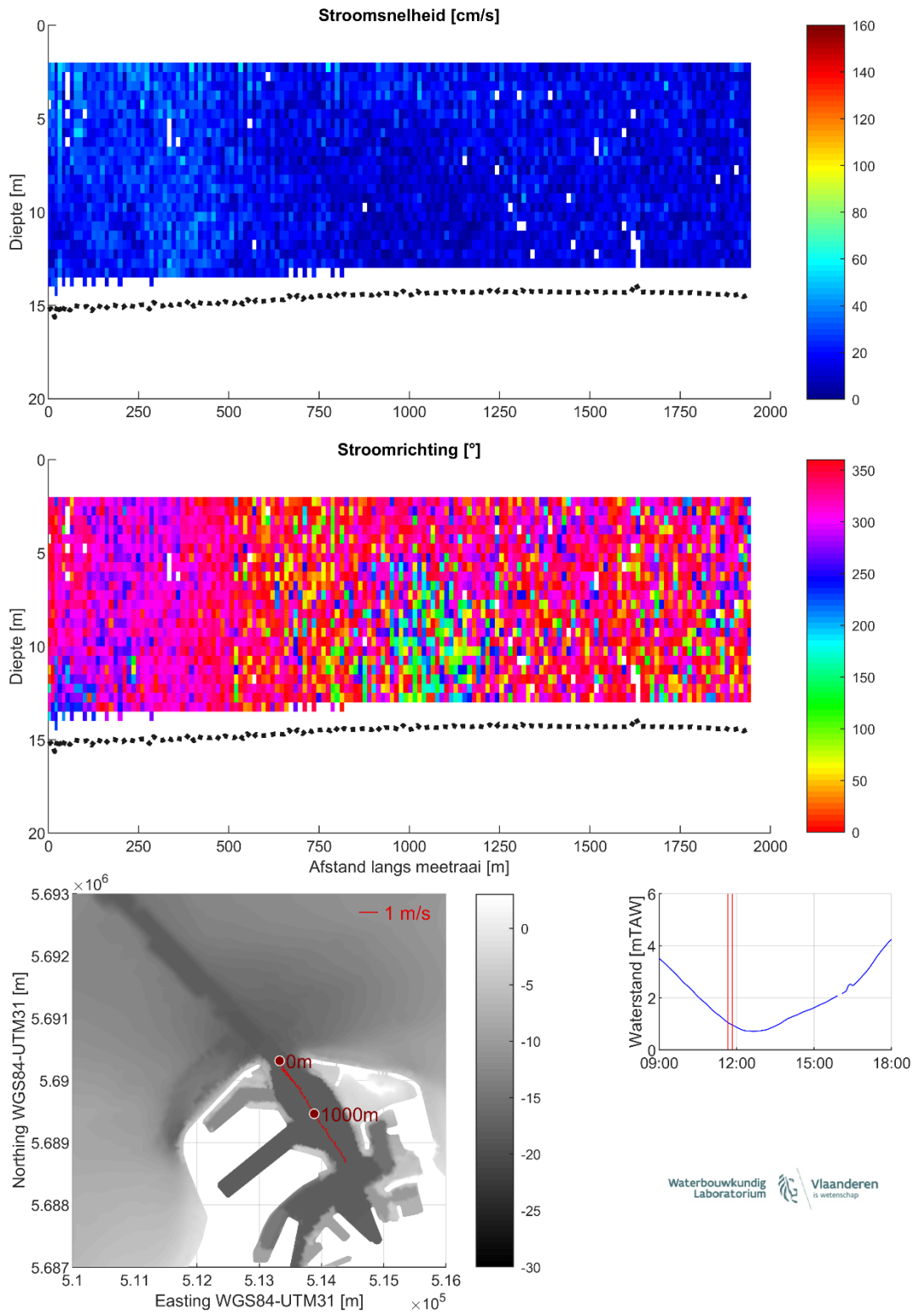
Figuur 19 – Stroomgegevens 07/08/2023 raai 14: snelheids grootte (top), -richting (midden) en diepte-gemiddelde vectoren (onder)
