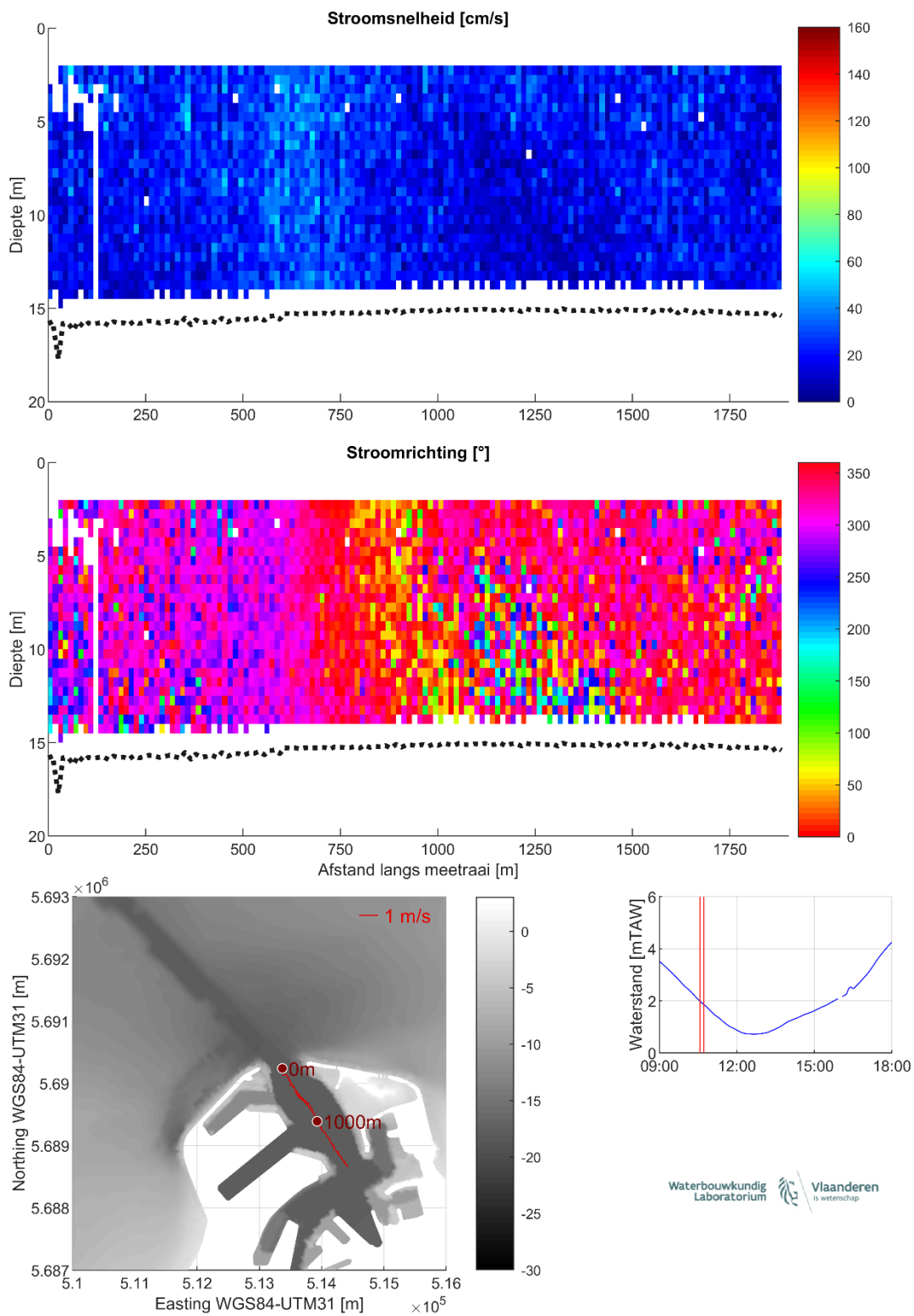
Figuur 13 – Stroomgegevens 07/08/2023 raai 8: snelheids grootte (top), -richting (midden) en diepte-gemiddelde vectoren (onder)
