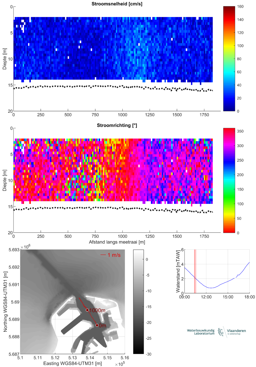
Figuur 12 – Stroomgegevens 07/08/2023 raai 7: snelheids grootte (top), -richting (midden) en diepte-gemiddelde vectoren (onder)
