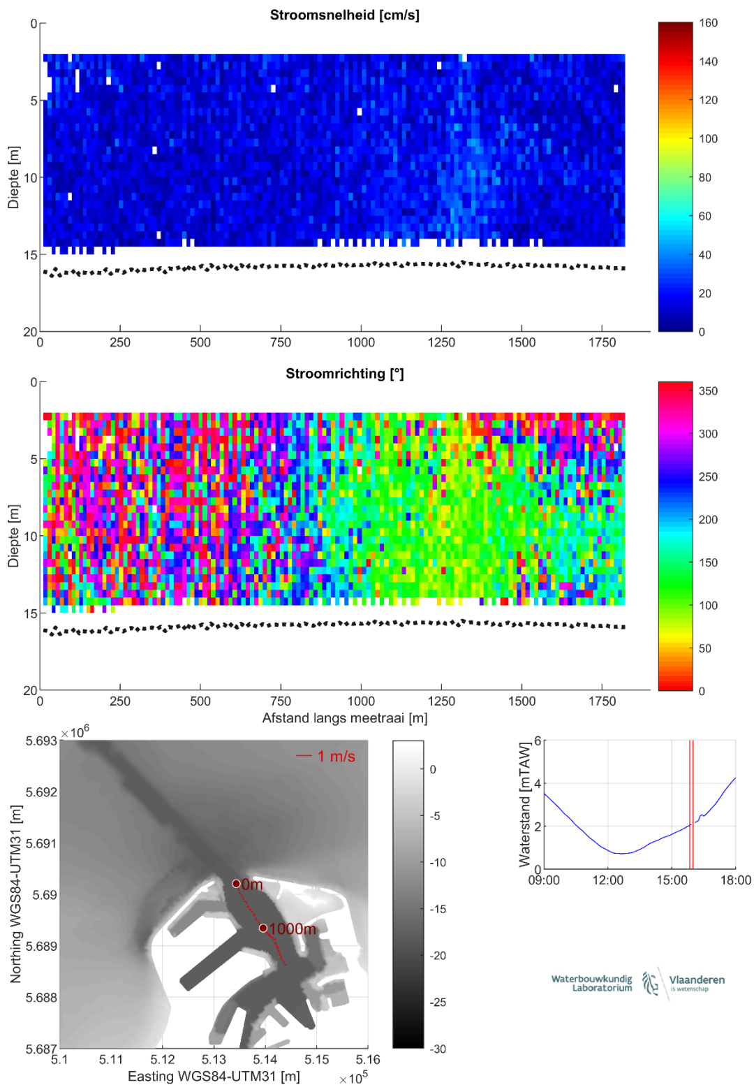
Figuur 41 – Stroomgegevens 07/08/2023 raai 36: snelheids grootte (top), -richting (midden) en diepte-gemiddelde vectoren (onder)
