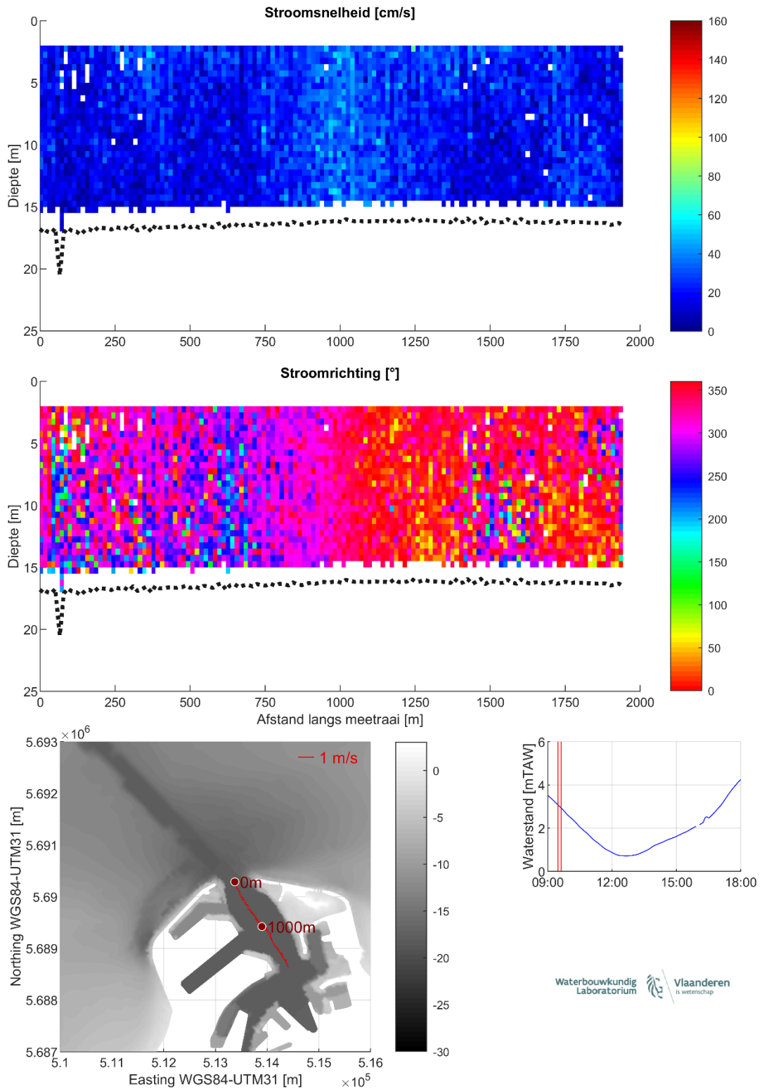
Figuur 7 – Stroomgegevens 07/08/2023 raai 2: snelheids grootte (top), -richting (midden) en diepte-gemiddelde vectoren (onder)
