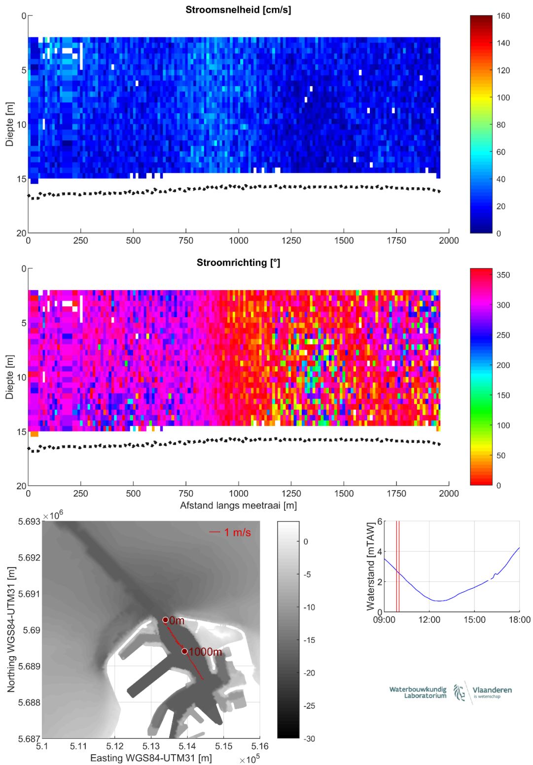
Figuur 9 – Stroomgegevens 07/08/2023 raai 4: snelheids grootte (top), -richting (midden) en diepte-gemiddelde vectoren (onder)
