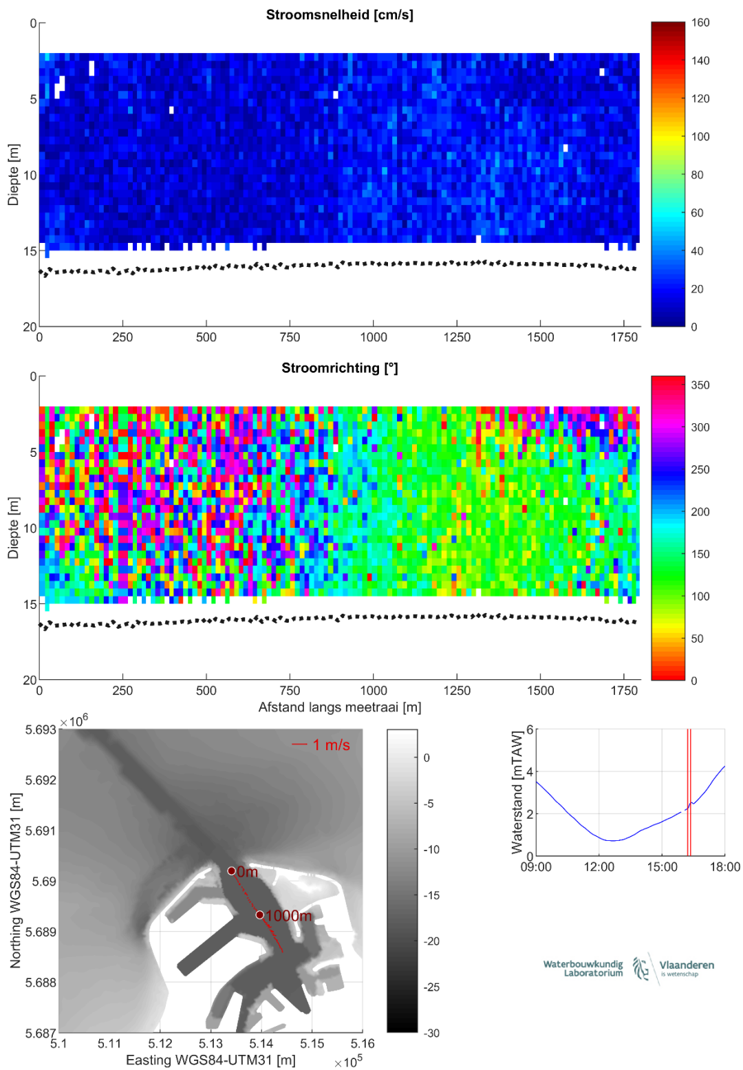
Figuur 43 – Stroomgegevens 07/08/2023 raai 38: snelheids grootte (top), -richting (midden) en diepte-gemiddelde vectoren (onder)
