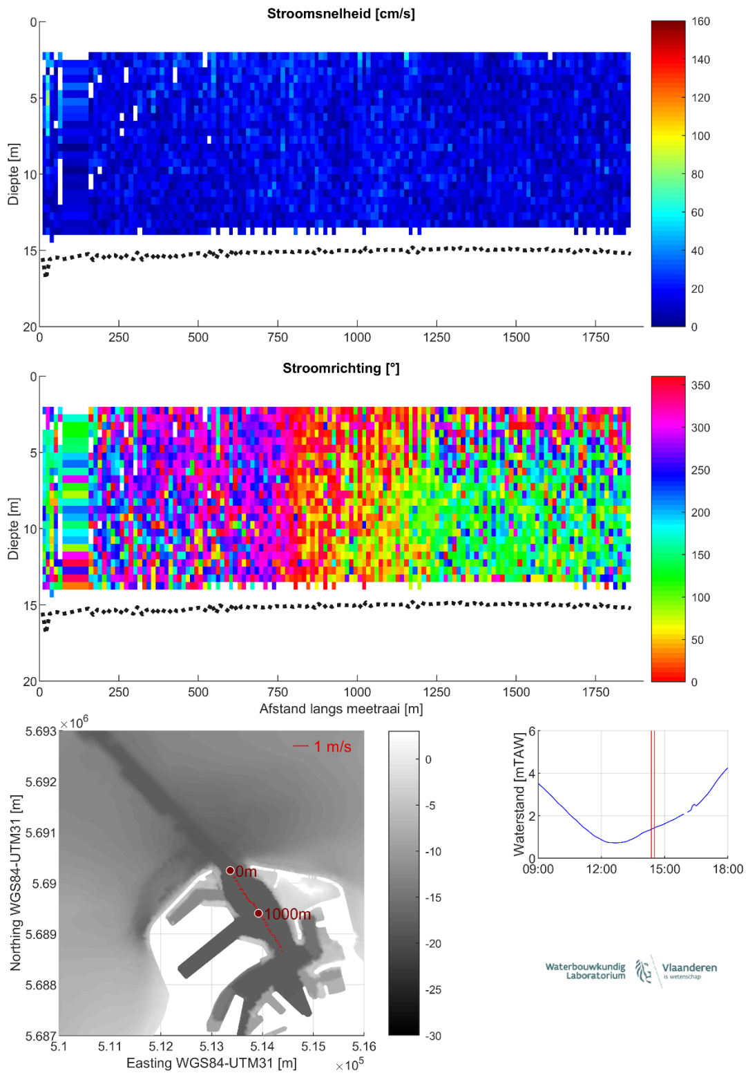
Figuur 33 – Stroomgegevens 07/08/2023 raai 28: snelheids grootte (top), -richting (midden) en diepte-gemiddelde vectoren (onder)
