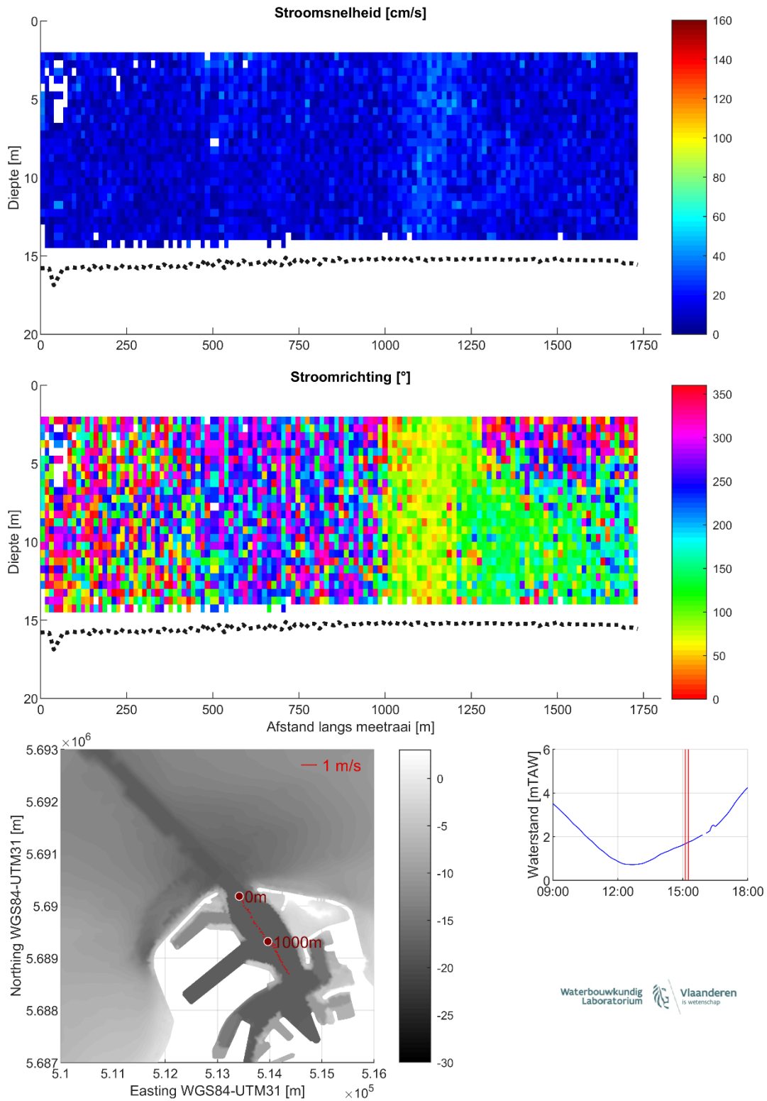
Figuur 37 – Stroomgegevens 07/08/2023 raai 32: snelheids grootte (top), -richting (midden) en diepte-gemiddelde vectoren (onder)
