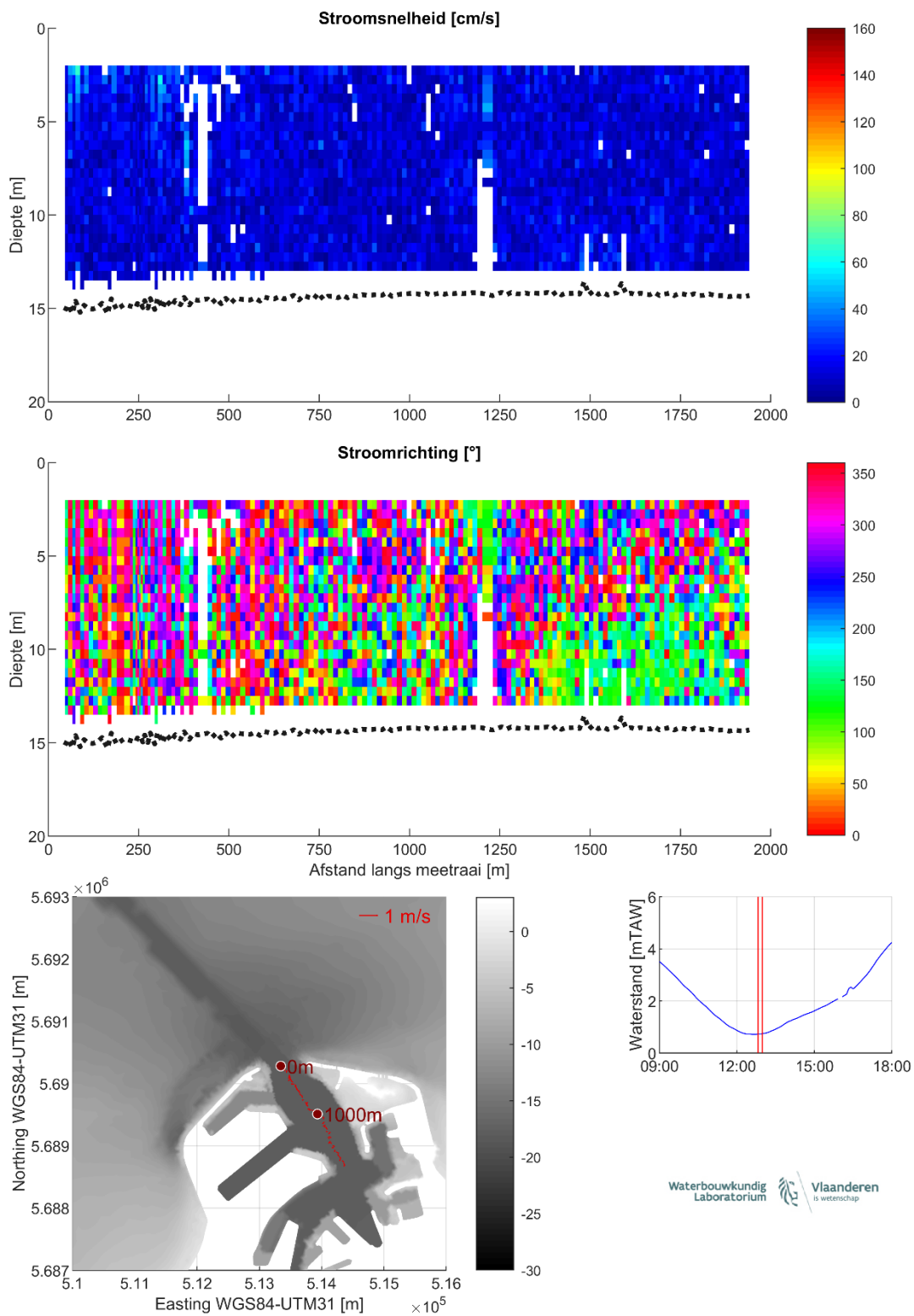
Figuur 25 – Stroomgegevens 07/08/2023 raai 20: snelheids grootte (top), -richting (midden) en diepte-gemiddelde vectoren (onder)
