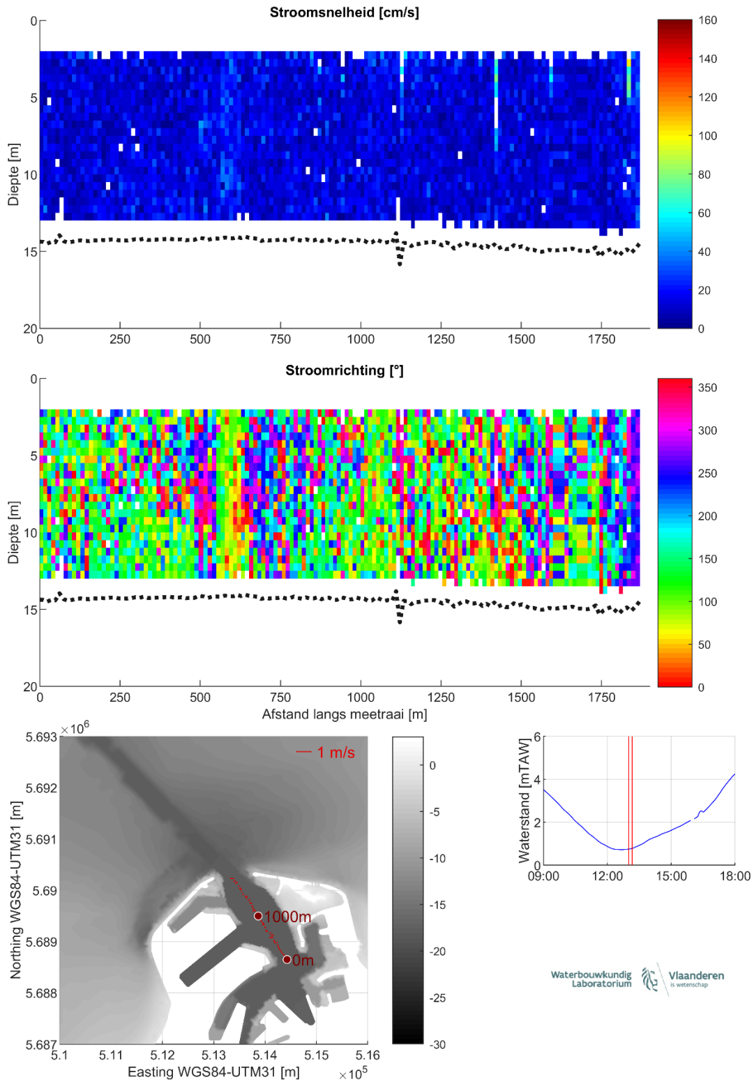
Figuur 26 – Stroomgegevens 07/08/2023 raai 21: snelheids grootte (top), -richting (midden) en diepte-gemiddelde vectoren (onder)
