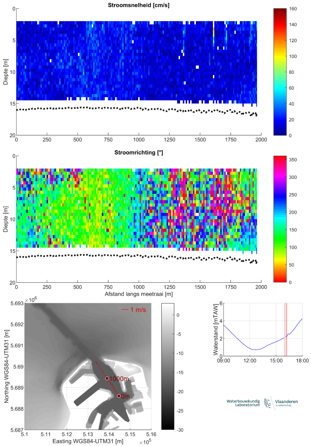
Figuur 42 – Stroomgegevens 07/08/2023 raai 37: snelheids grootte (top), -richting (midden) en diepte-gemiddelde vectoren (onder)
