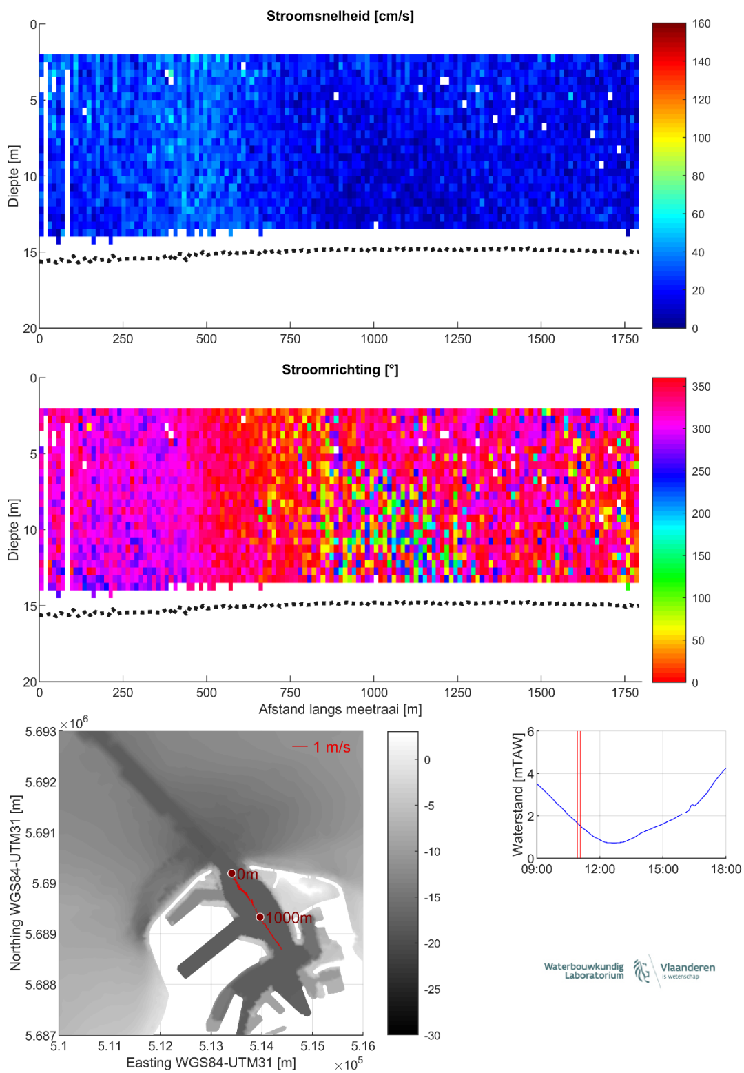
Figuur 15 – Stroomgegevens 07/08/2023 raai 10: snelheids grootte (top), -richting (midden) en diepte-gemiddelde vectoren (onder)
