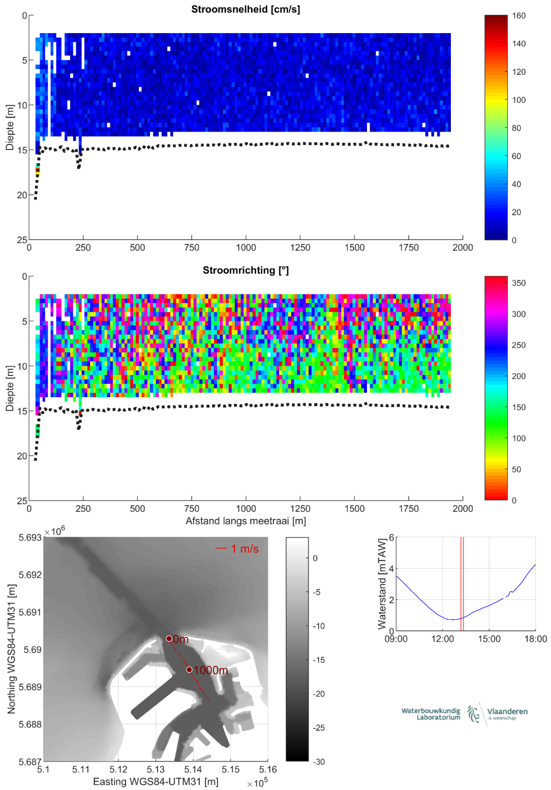
Figuur 27 – Stroomgegevens 07/08/2023 raai 22: snelheids grootte (top), -richting (midden) en diepte-gemiddelde vectoren (onder)
