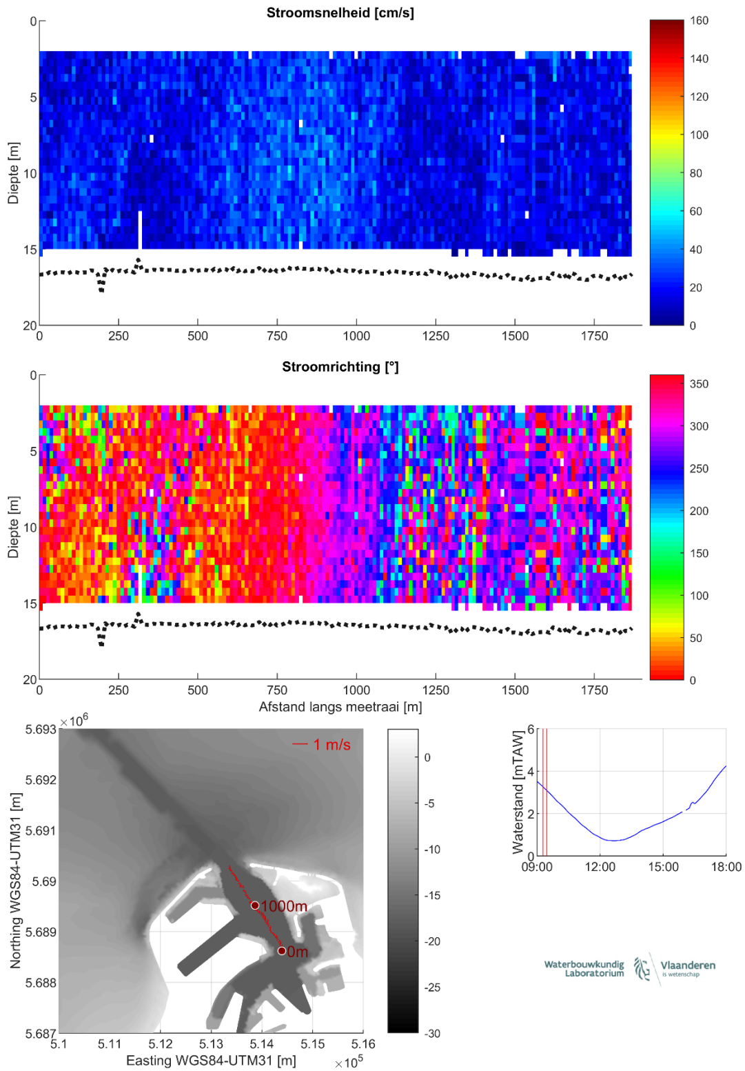
Figuur 6 – Stroomgegevens 07/08/2023 raai 1: snelheids grootte (top), -richting (midden) en diepte-gemiddelde vectoren (onder)
