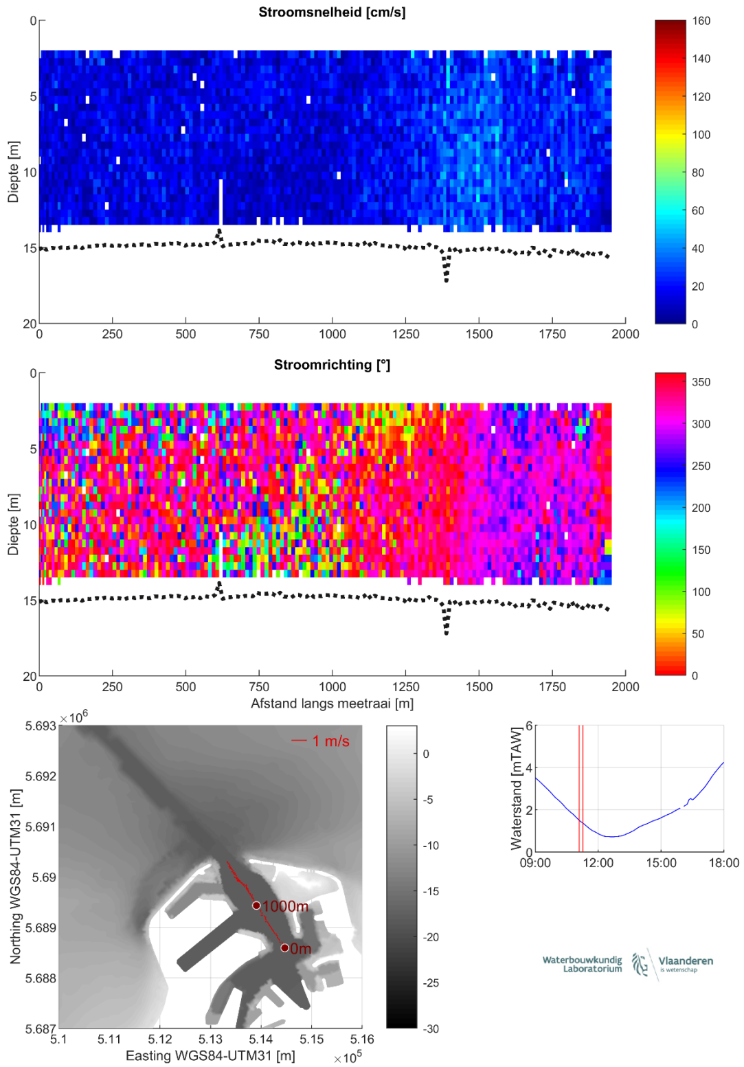
Figuur 16 – Stroomgegevens 07/08/2023 raai 11: snelheids grootte (top), -richting (midden) en diepte-gemiddelde vectoren (onder)
