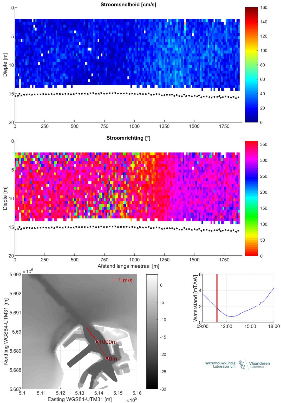
Figuur 14 – Stroomgegevens 07/08/2023 raai 9: snelheids grootte (top), -richting (midden) en diepte-gemiddelde vectoren (onder)
