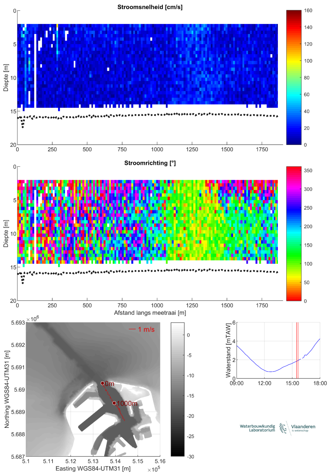
Figuur 39 – Stroomgegevens 07/08/2023 raai 34: snelheids grootte (top), -richting (midden) en diepte-gemiddelde vectoren (onder)
