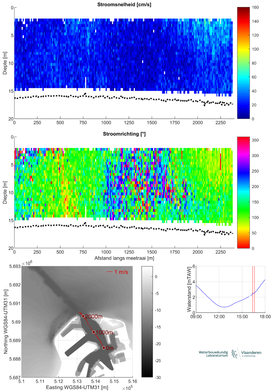
Figuur 44 – Stroomgegevens 07/08/2023 raai 39: snelheidsgrootte (top), -richting (midden) en diepte-gemiddelde vectoren (onder)
