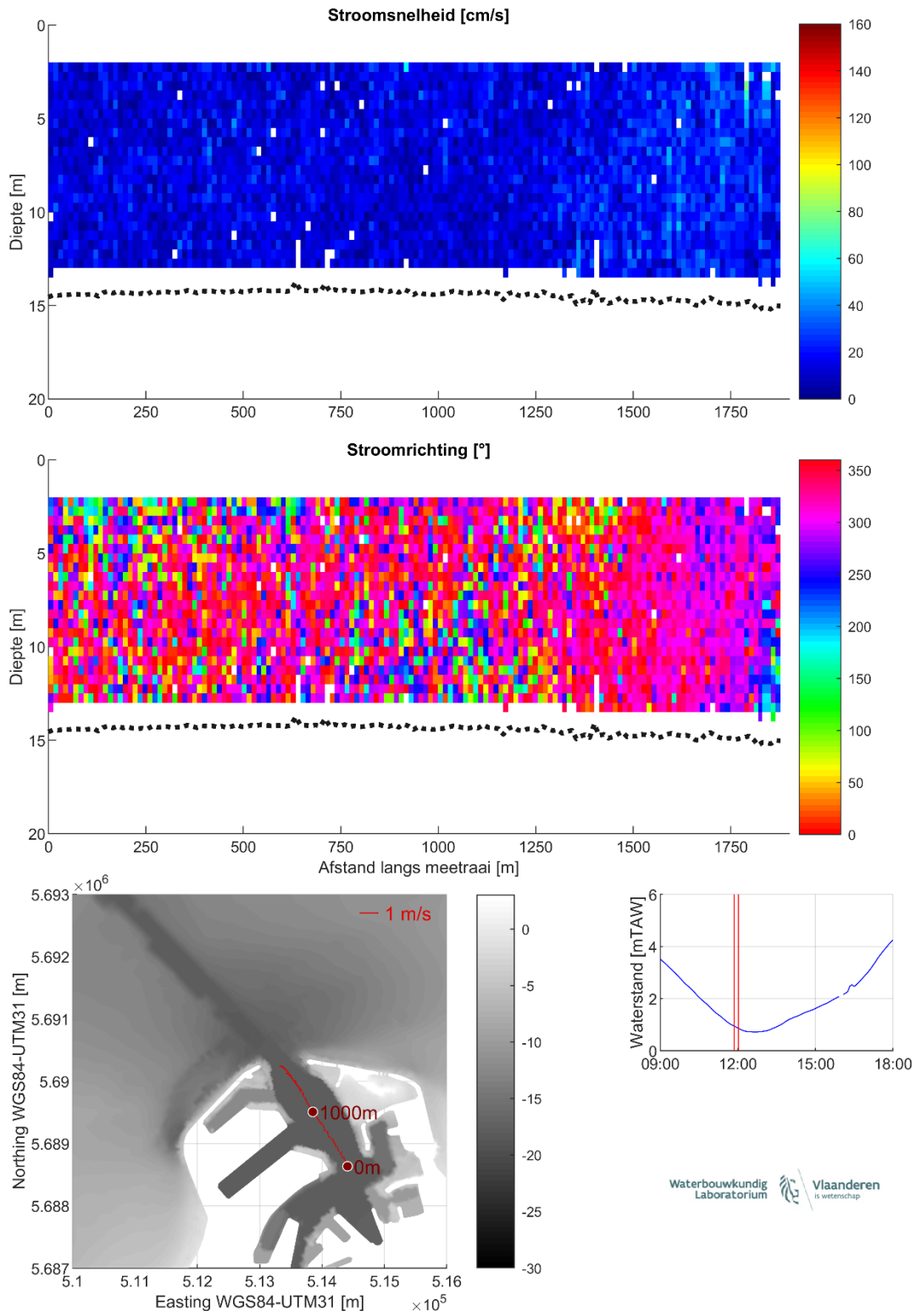
Figuur 20 – Stroomgegevens 07/08/2023 raai 15: snelheids grootte (top), -richting (midden) en diepte-gemiddelde vectoren (onder)
