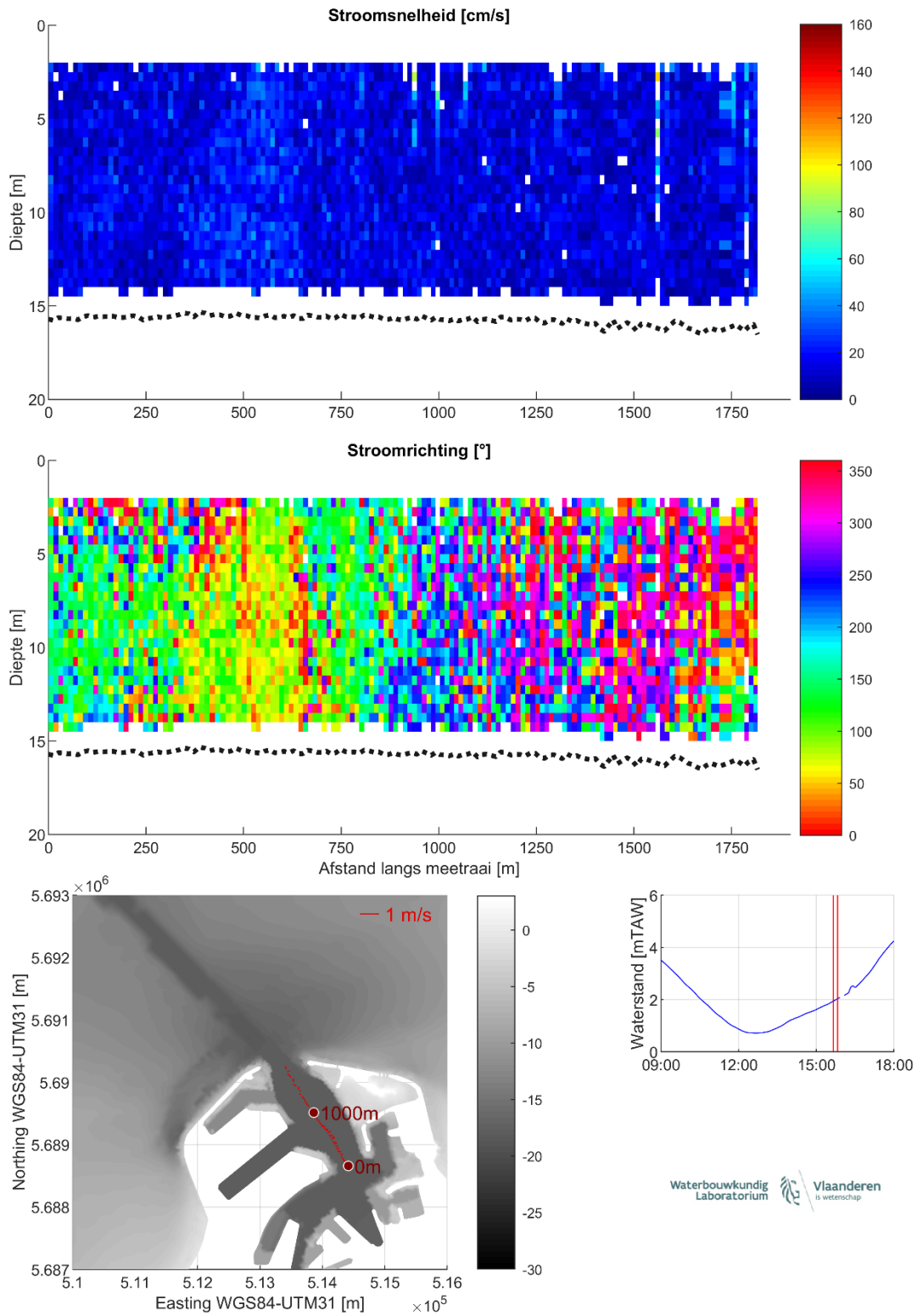
Figuur 40 – Stroomgegevens 07/08/2023 raai 35: snelheids grootte (top), -richting (midden) en diepte-gemiddelde vectoren (onder)
