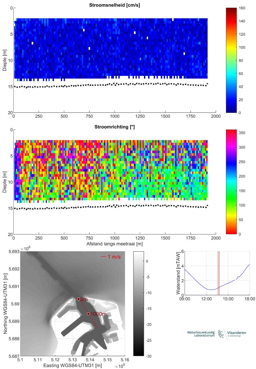
Figuur 29 – Stroomgegevens 07/08/2023 raai 24: snelheids grootte (top), -richting (midden) en diepte-gemiddelde vectoren (onder)
