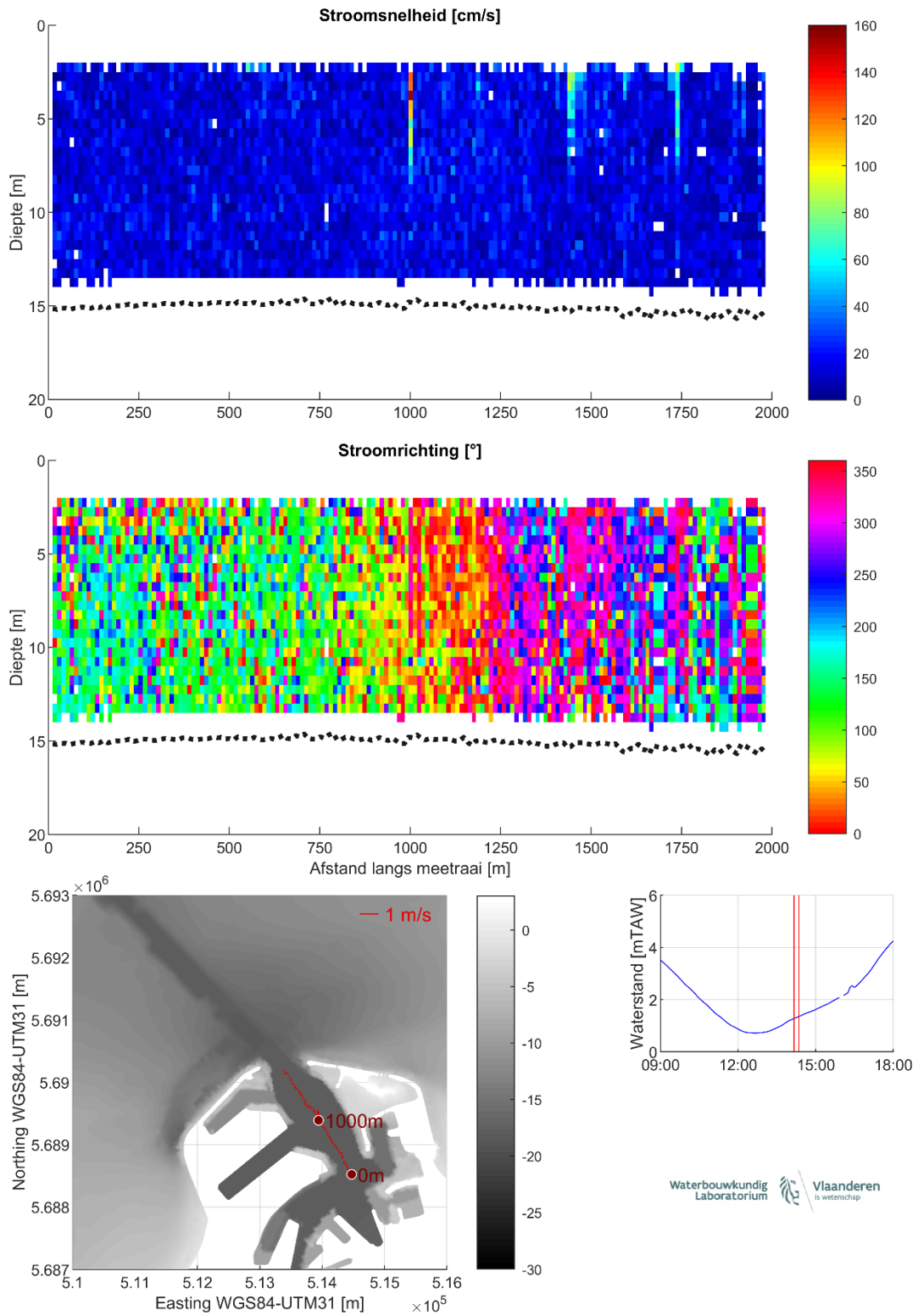
Figuur 32 – Stroomgegevens 07/08/2023 raai 27: snelheids grootte (top), -richting (midden) en diepte-gemiddelde vectoren (onder)
