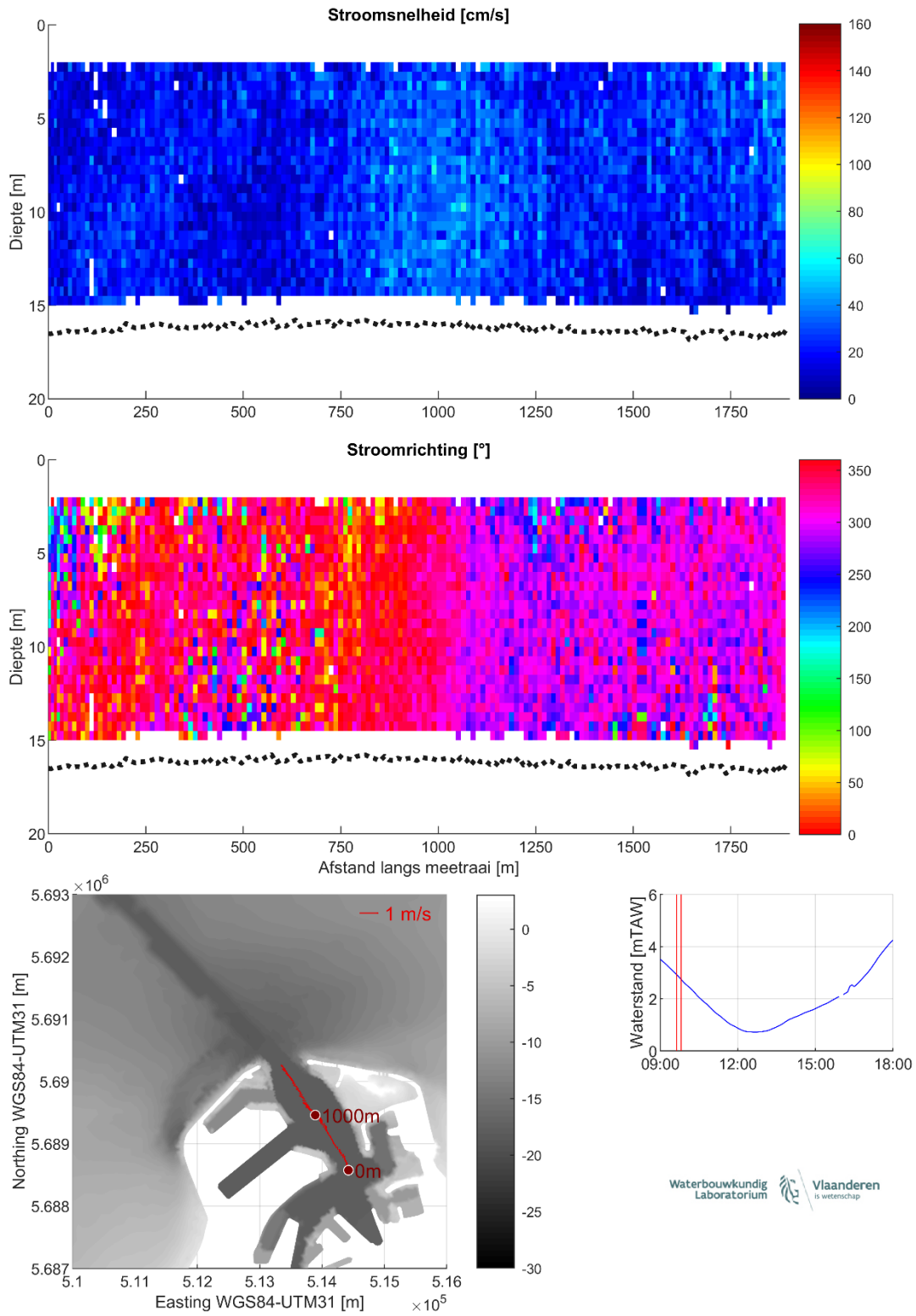
Figuur 8 – Stroomgegevens 07/08/2023 raai 3: snelheidsgrootte (top), -richting (midden) en diepte-gemiddelde vectoren (onder)
