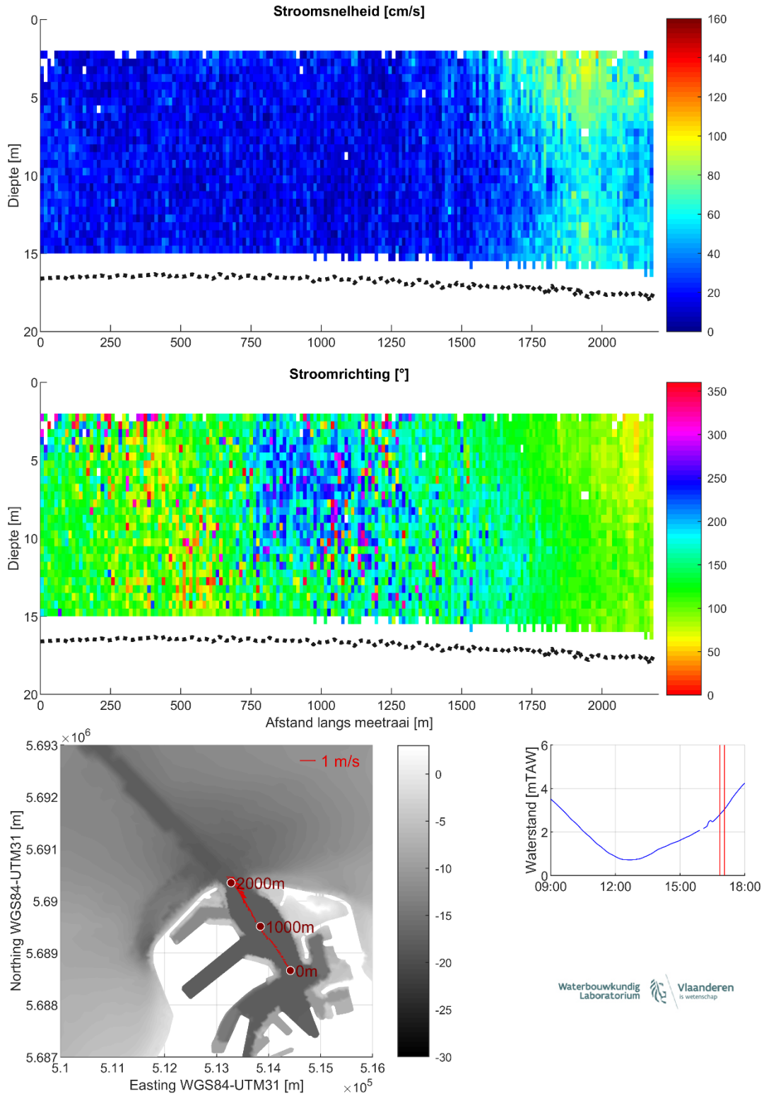
Figuur 46 – Stroomgegevens 07/08/2023 raai 41: snelheids grootte (top), -richting (midden) en diepte-gemiddelde vectoren (onder)
