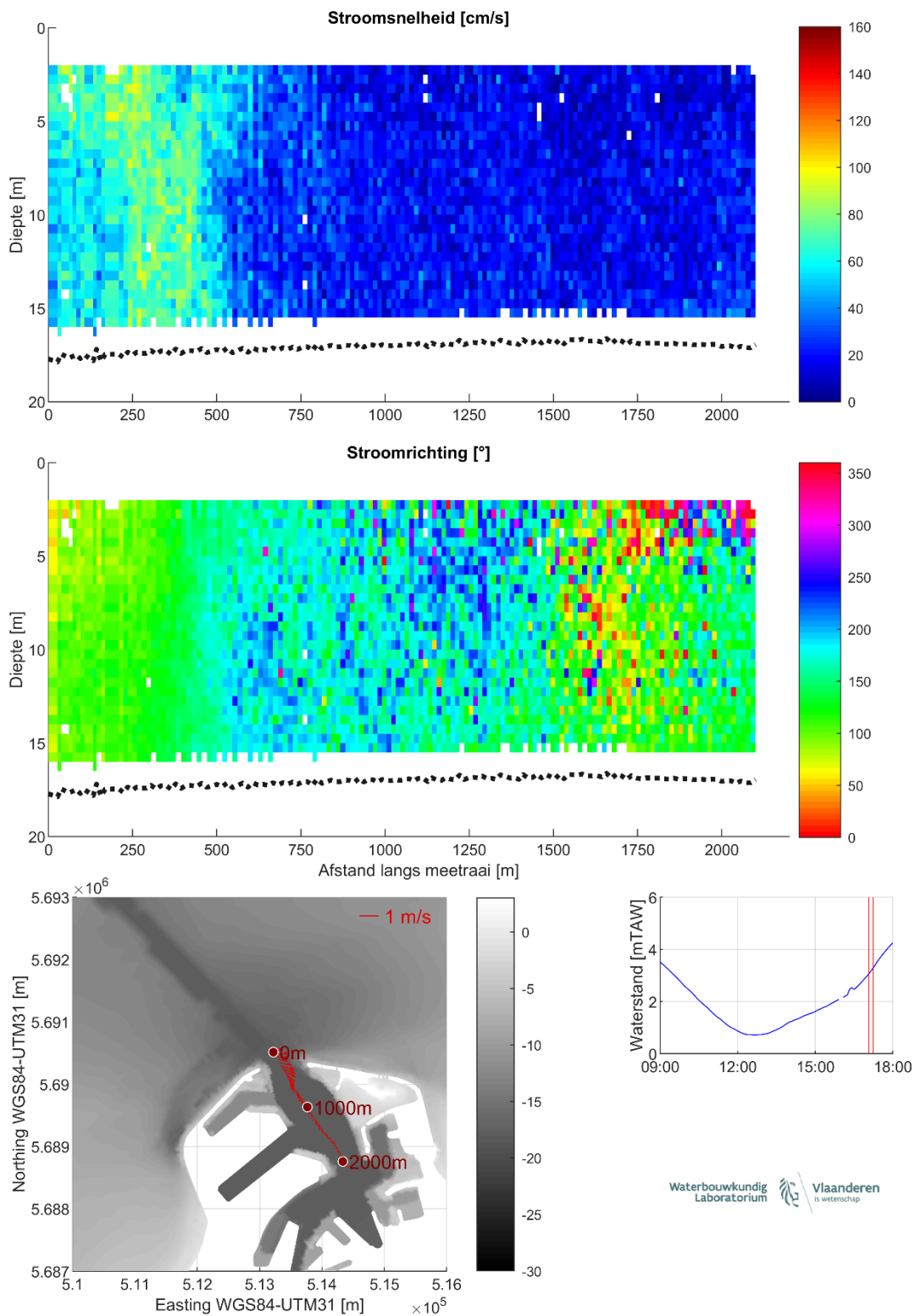
Figuur 47 – Stroomgegevens 07/08/2023 raai 42: snelheids grootte (top), -richting (midden) en diepte-gemiddelde vectoren (onder)
