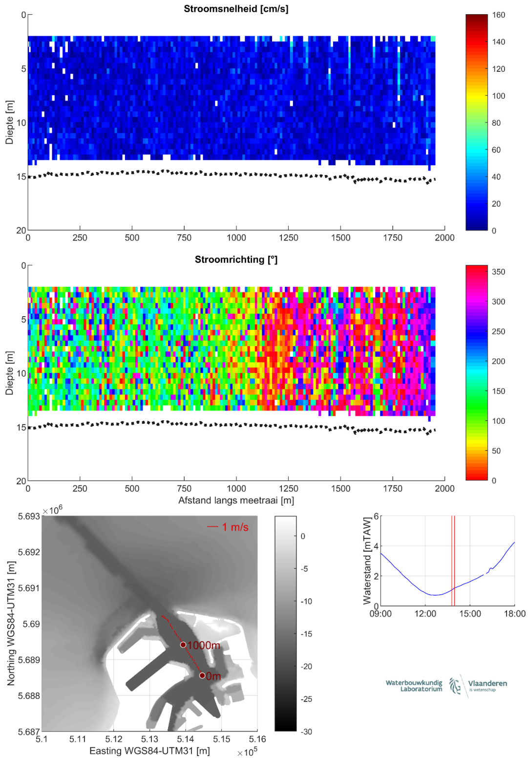
Figuur 30 – Stroomgegevens 07/08/2023 raai 25: snelheids grootte (top), -richting (midden) en diepte-gemiddelde vectoren (onder)
