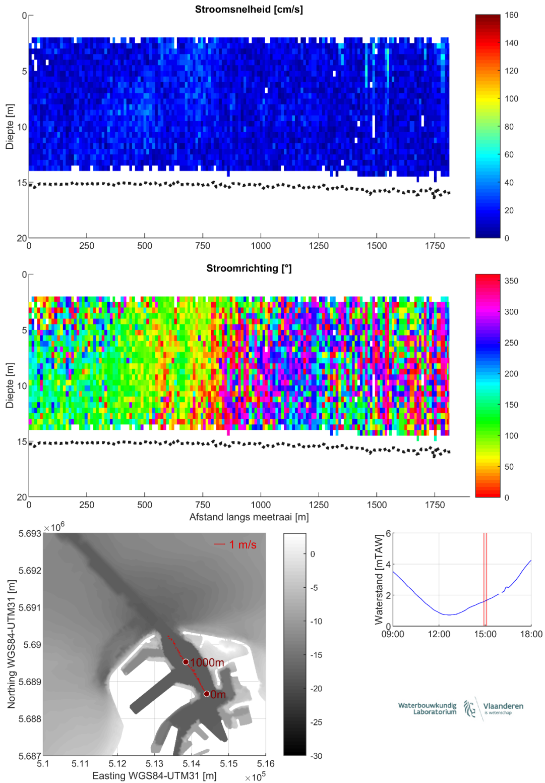
Figuur 36 – Stroomgegevens 07/08/2023 raai 31: snelheids grootte (top), -richting (midden) en diepte-gemiddelde vectoren (onder)
