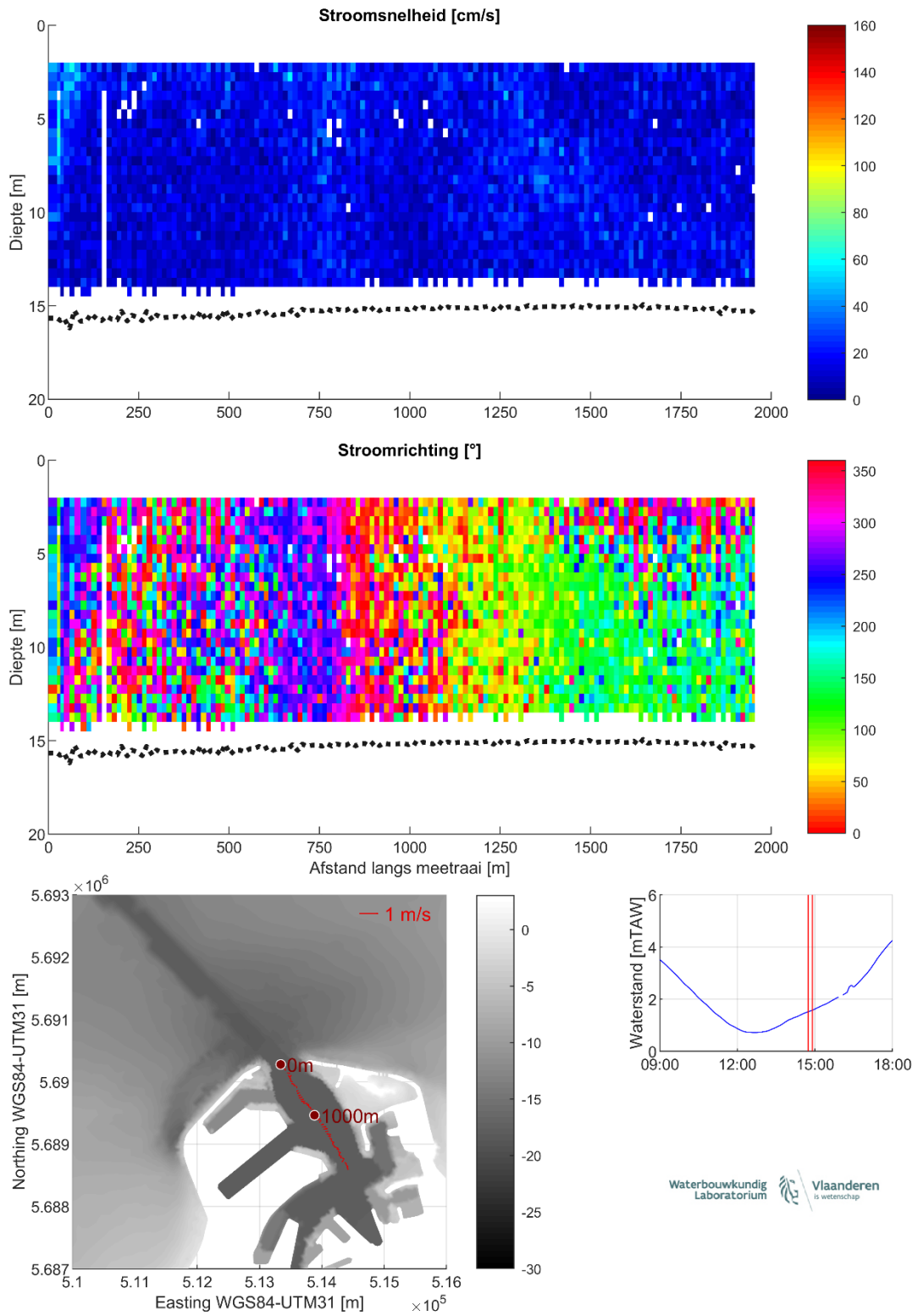
Figuur 35 – Stroomgegevens 07/08/2023 raai 30: snelheids grootte (top), -richting (midden) en diepte-gemiddelde vectoren (onder)
