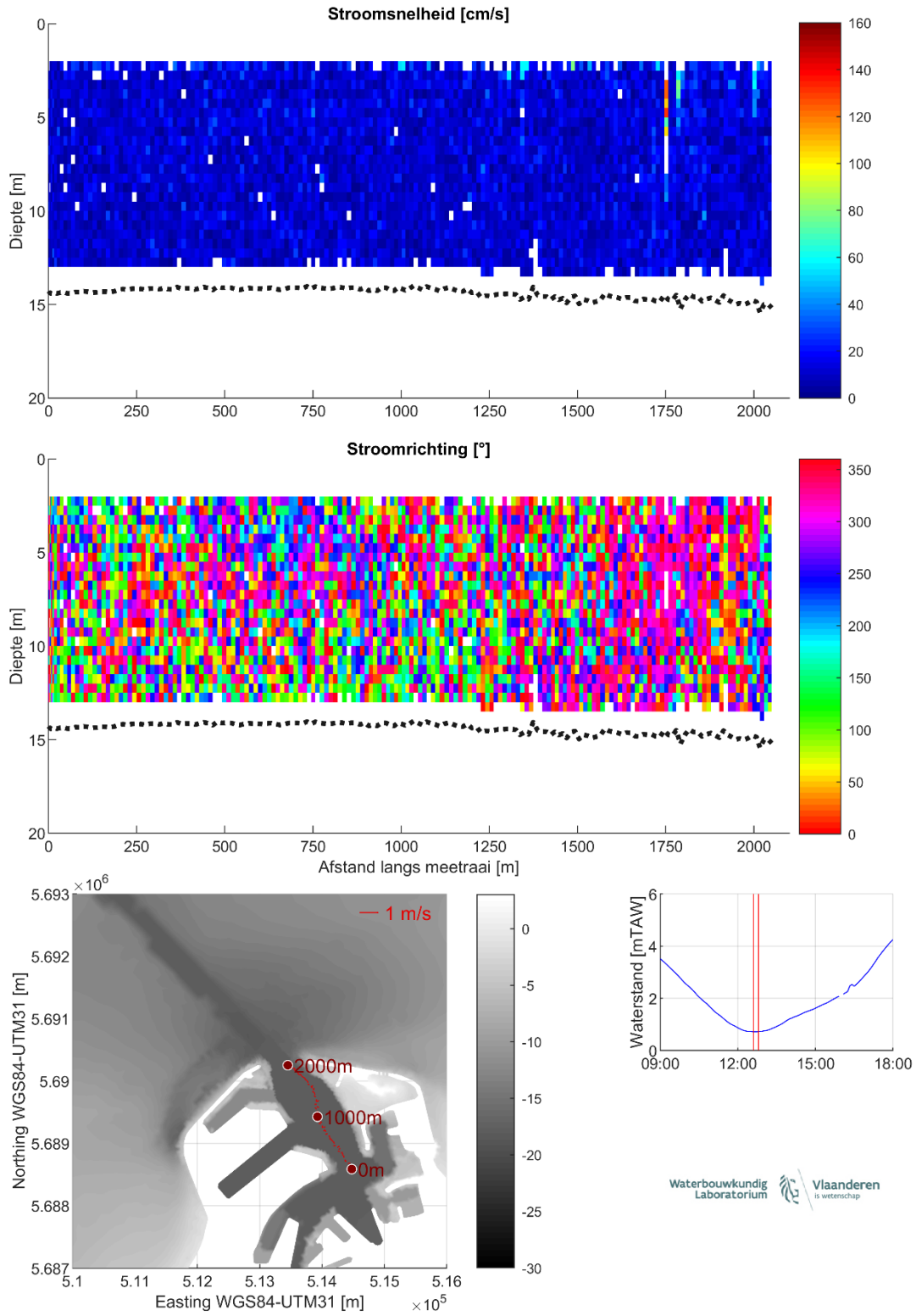
Figuur 24 – Stroomgegevens 07/08/2023 raai 19: snelheids grootte (top), -richting (midden) en diepte-gemiddelde vectoren (onder)
