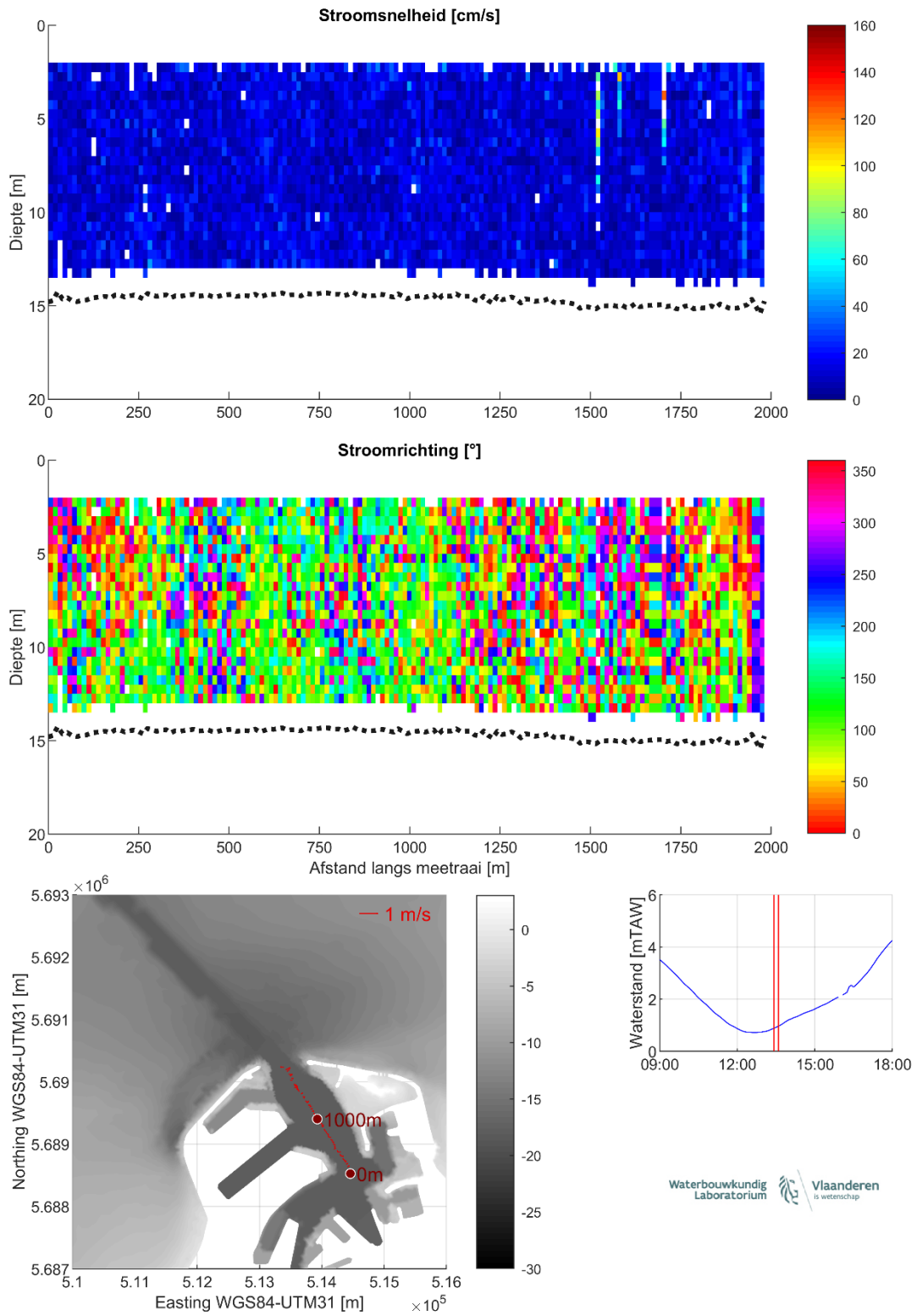
Figuur 28 – Stroomgegevens 07/08/2023 raai 23: snelheids grootte (top), -richting (midden) en diepte-gemiddelde vectoren (onder)
