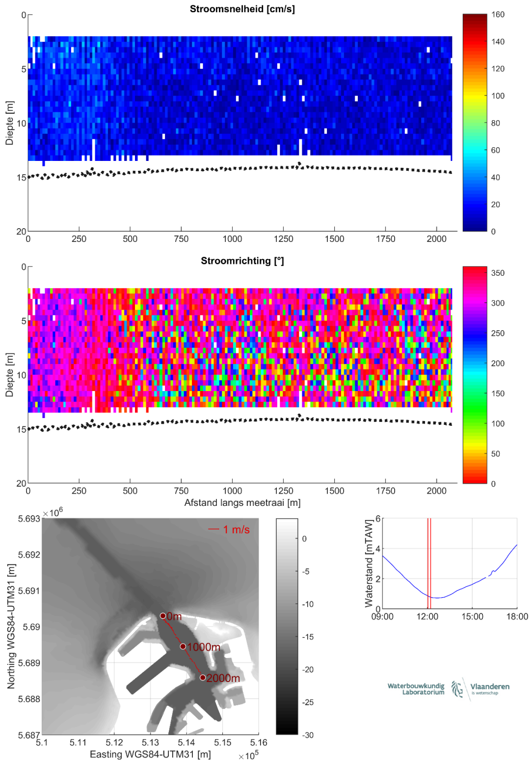
Figuur 21 – Stroomgegevens 07/08/2023 raai 16: snelheids grootte (top), -richting (midden) en diepte-gemiddelde vectoren (onder)
