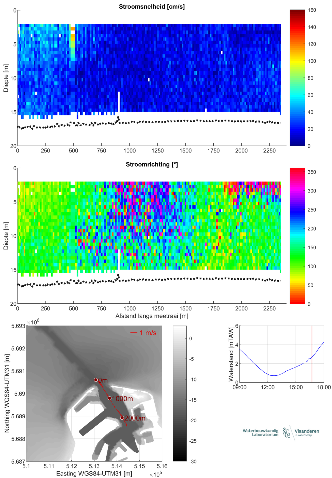
Figuur 45 – Stroomgegevens 07/08/2023 raai 40: snelheids grootte (top), -richting (midden) en diepte-gemiddelde vectoren (onder)
