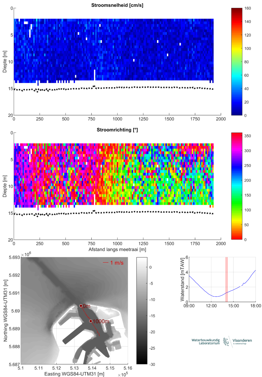
Figuur 31 – Stroomgegevens 07/08/2023 raai 26: snelheids grootte (top), -richting (midden) en diepte-gemiddelde vectoren (onder)
