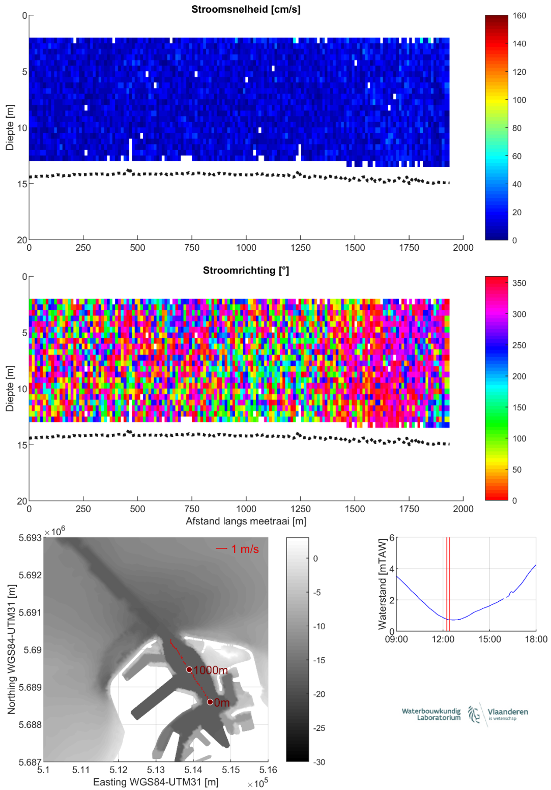
Figuur 22 – Stroomgegevens 07/08/2023 raai 17: snelheids grootte (top), -richting (midden) en diepte-gemiddelde vectoren (onder)
