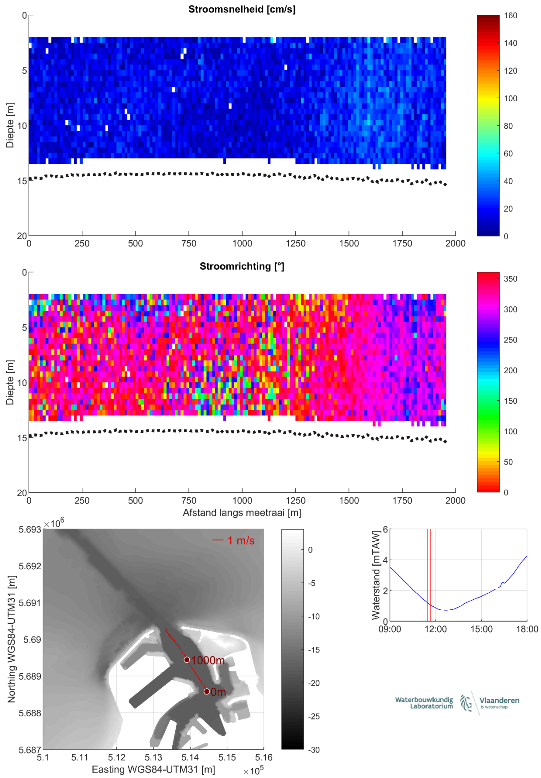
Figuur 18 – Stroomgegevens 07/08/2023 raai 13: snelheids grootte (top), -richting (midden) en diepte-gemiddelde vectoren (onder)
